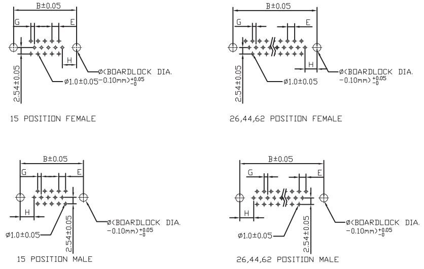
P.C.B LAYOUT PATTERN
