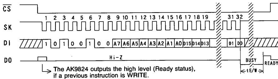
WRITE (AK9824)
