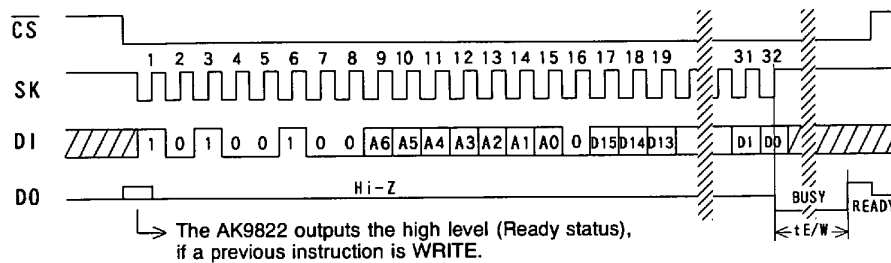
WRITE (AK9822)
