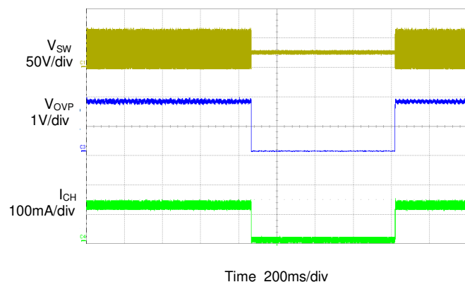
VOU Short/Diode Open Protection
