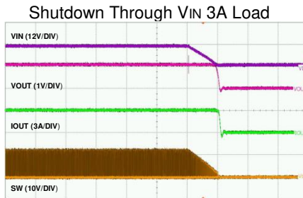
Time-200μs/div
