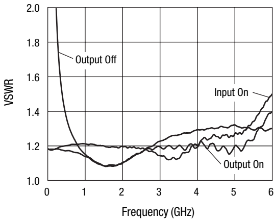
VSWR, 85 °C V_{DD} = 5\text{ V}, V_{CTL} = 0/5\text{ V}
