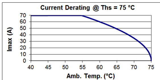
B25620B1367K203
