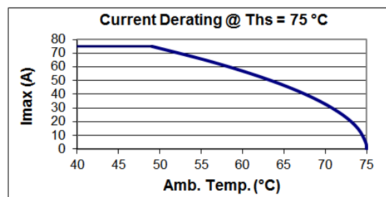
B25620B1577K203
