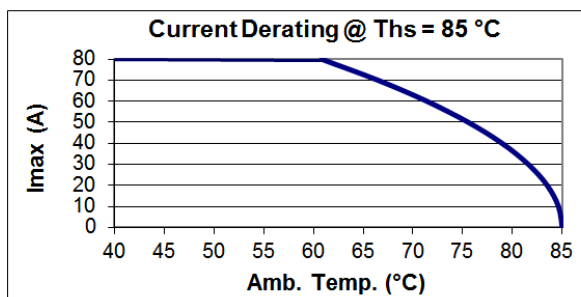
B25620B1487K101
