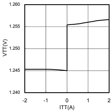
Fig.7 ITT-VTT (DDR1)
