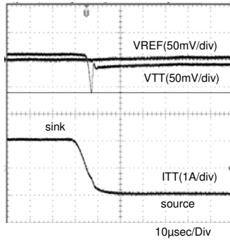
Fig.2 DDR3 (1A→-1A)
