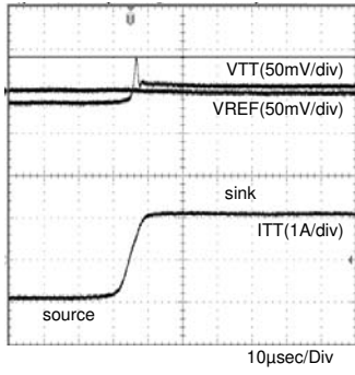
Fig.1 DDR3 (-1A→1A)
