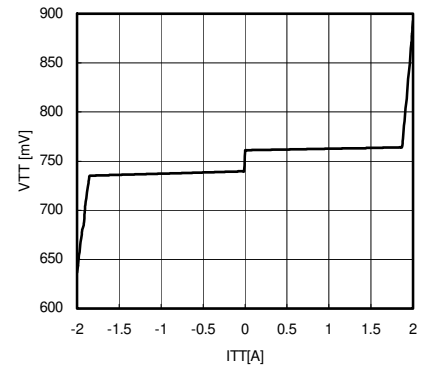
Fig.6 ITT-VTT (DDR3)
