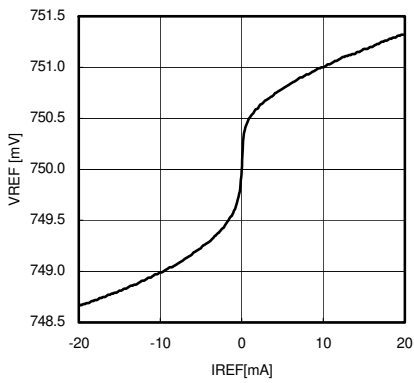
Fig.7 IREF-VREF (DDR3)
