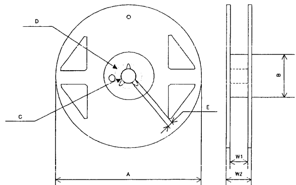
Fig. 4 Reel dimensions
