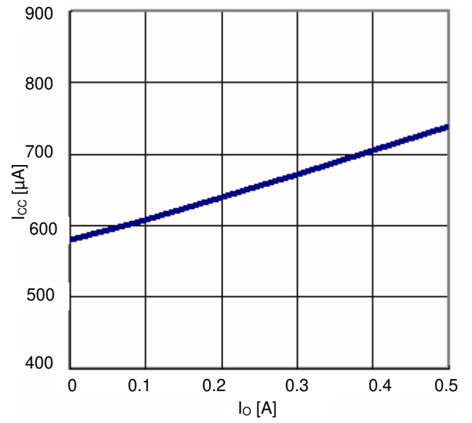
Fig.20 I_o - I_{cc}
