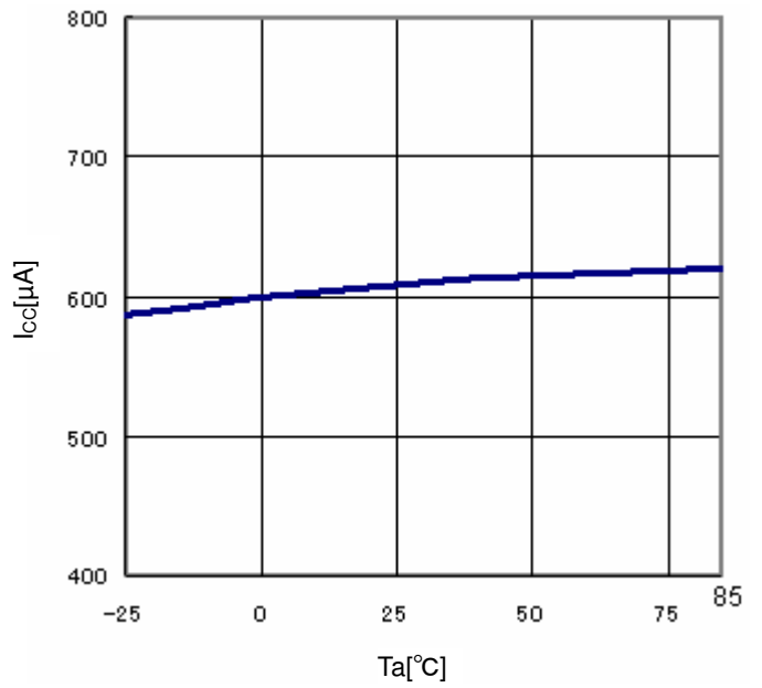
Fig.9 T_a-I_{cc}
