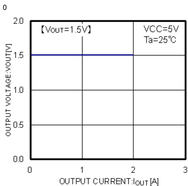
Fig.6 Iout-Vout
