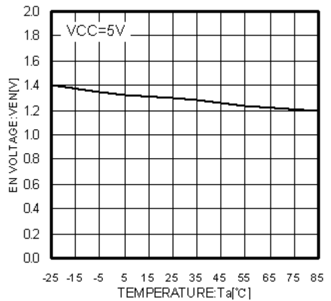
Fig.11 Ta-VEN
