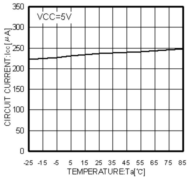
Fig.12 T_a - I_{cc}
