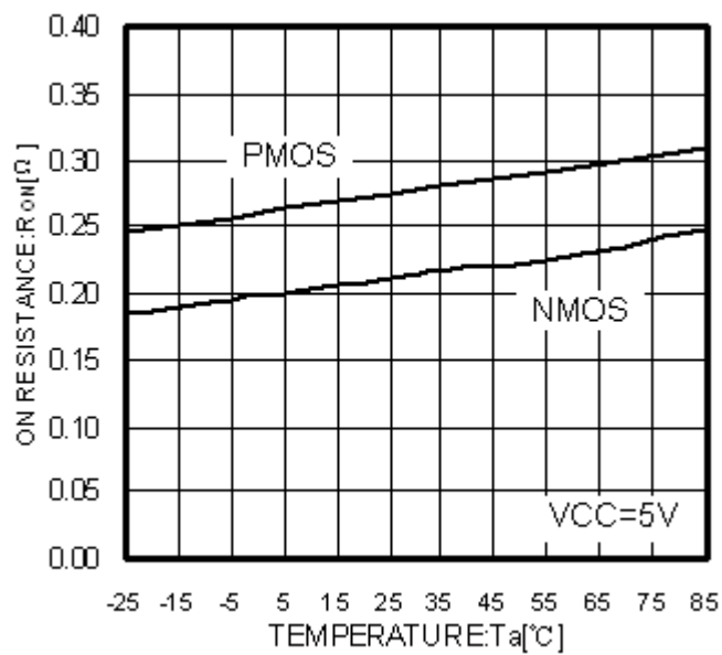
Fig.10 Ta-RONN, RONP
