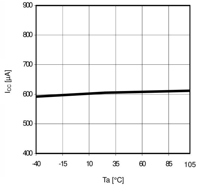
Fig. 22 T_a - I_{cc}
