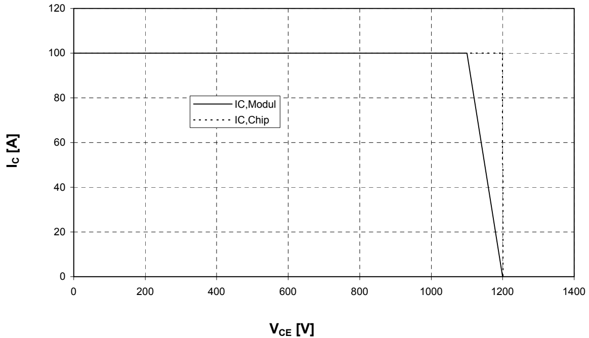
Sicherer Arbeitsbereich Wechselr. (RBSOA) I_c = f(V_{CE}) Reverse bias safe operating area Inverter (RBSOA) T_{vj} = 125^\circ C, V_{GE} = \pm 15V, R_G = 15 \text{ Ohm}
