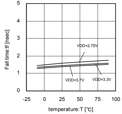
Fig.81 48MHz
