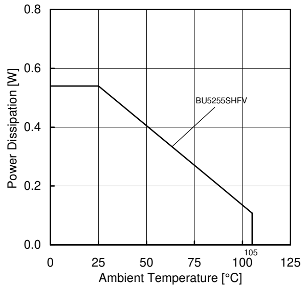
(d) BU5255SHFV
