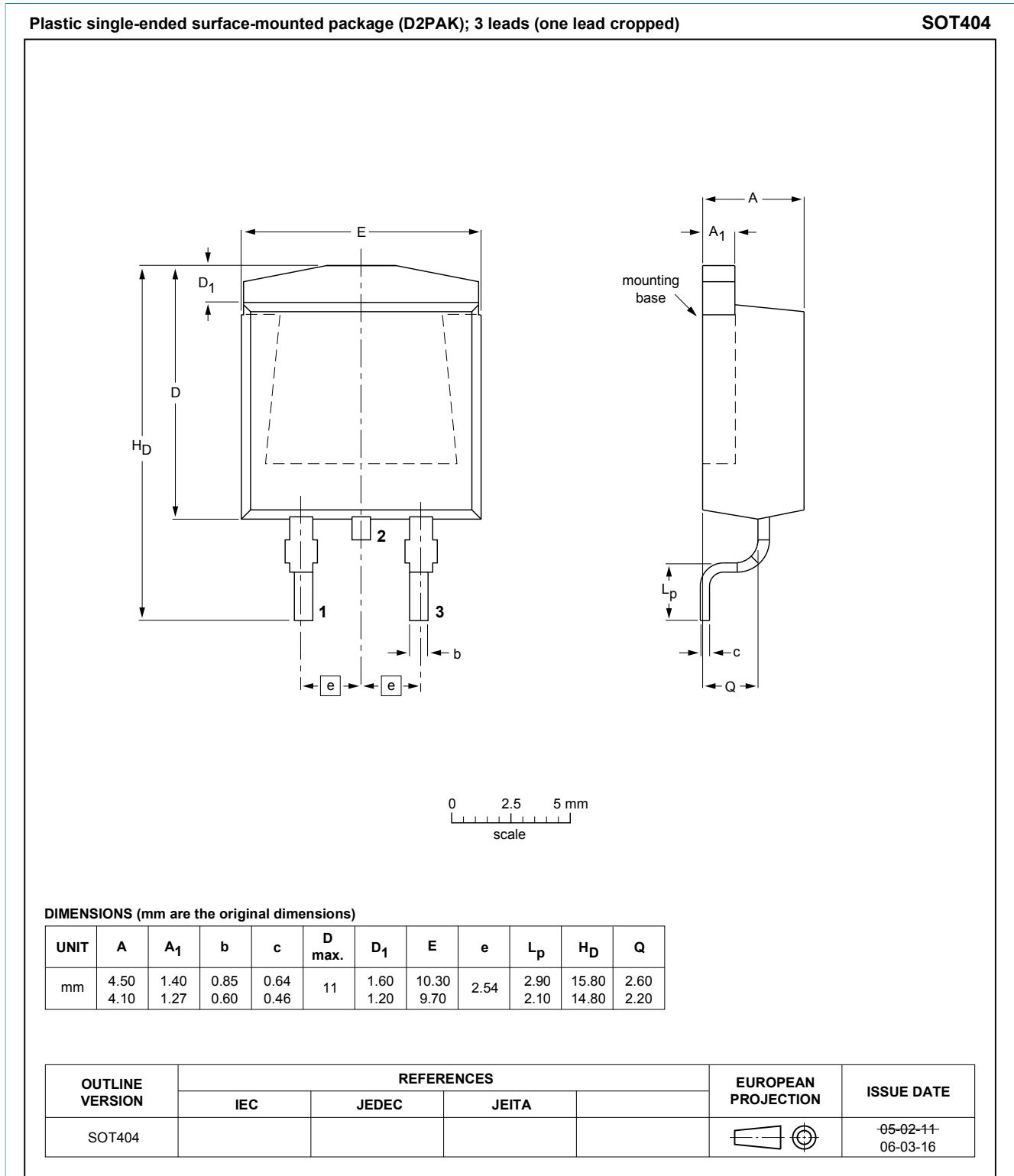
Fig. 16. D2PAK (SOT404)
