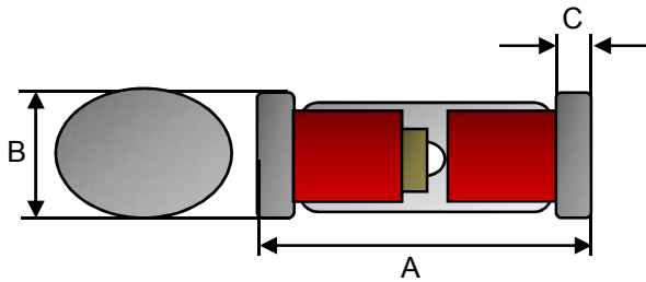
Mini-MELF
