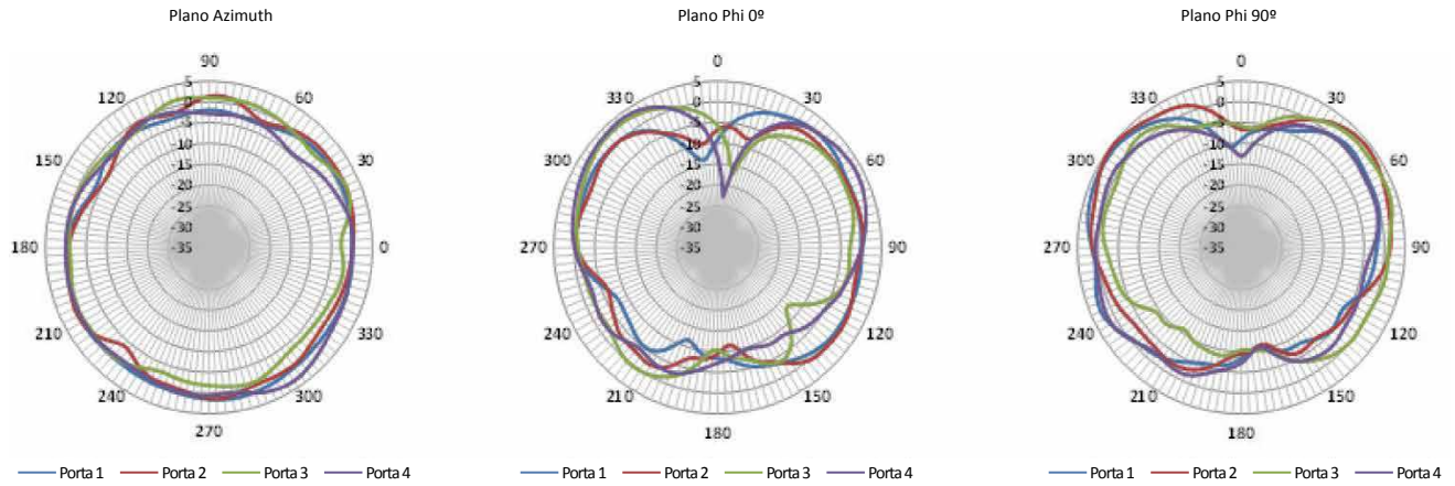
Diagrama de Radiação em 4900 MHz
