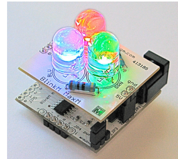
BlinkM MaxM
