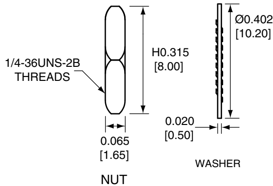
NUT
