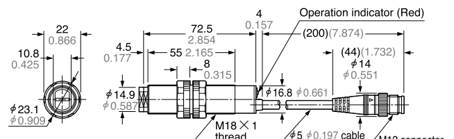
CY-19-J Sensor
