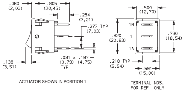
D102J12S215QA SPDT
