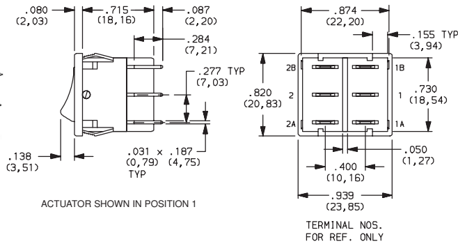
D201J12S215QA DPDT
