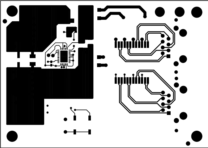
Layer 1. Top Layer
