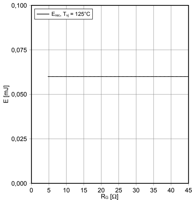
Schaltverluste Diode-Chopper (typisch) switching losses Diode-Chopper (typical) E_{rec} = f(R_G) I_F = 30 A, V_{CE} = 600 V
