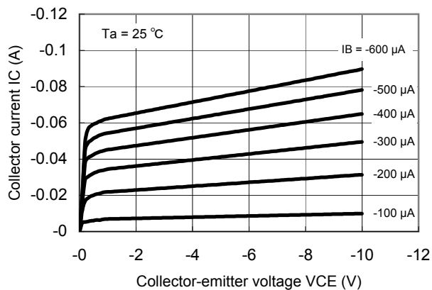
IC - VCE
