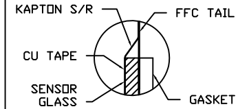
SECTION A-A SCALE: 8/1
