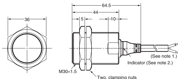
E2AU-M30KS15-WP-□□
