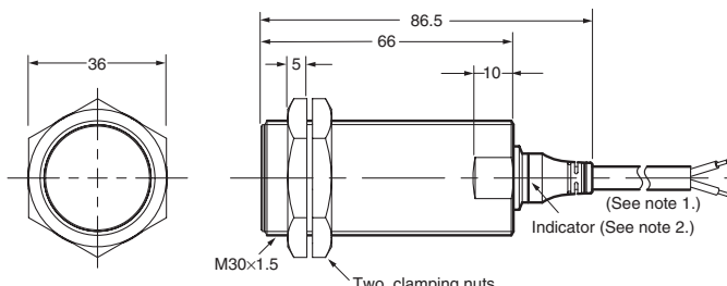
E2AU-M30LS15-WP-□□
