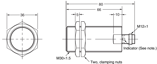
E2AU-M30LS15-M1-□□
