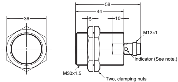
E2AU-M30KS15-M1-□□
