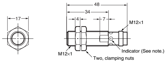
E2AU-M12KS04-M1-□□
