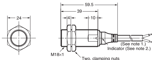
E2AU-M18KS08-WP-□□
