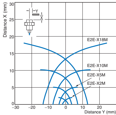
E2E-X□ME□/-X□MY□/-X□MF□
