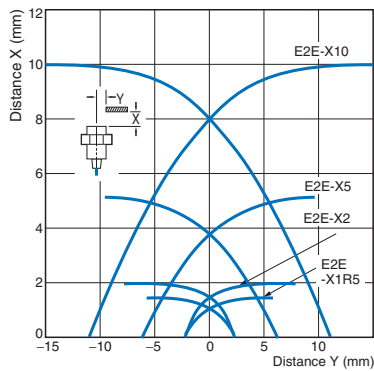
E2E-X□E□/-X□Y□/-X□F□
