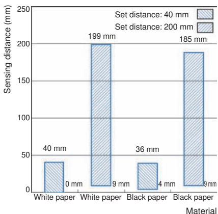
E3Z-LS□1/LS□6
