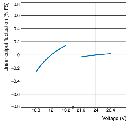
E8CC-AN0C
