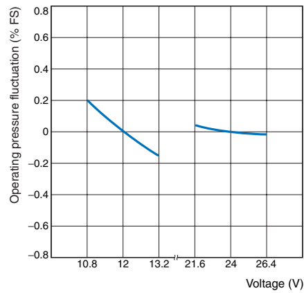
E8CC-AN0C
