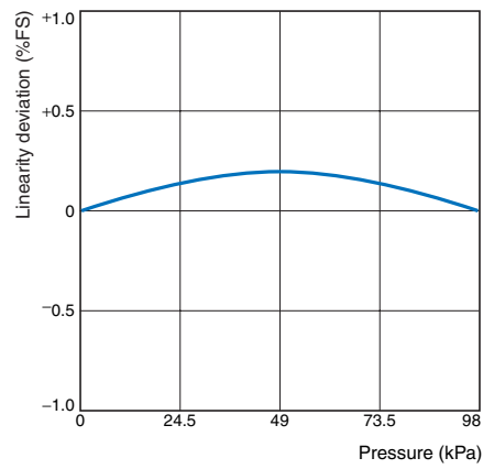
E8CC-A01C
