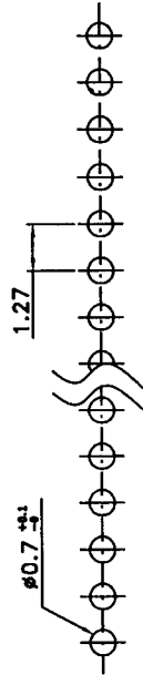
P.C.B LAYOUT
