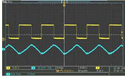
Vin=10V Vout=5V Iout=1A
