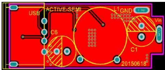
TOP LAYER
