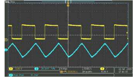
Vin=10V Vout=5V Iout=2.4A
