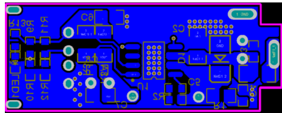
BOTTOM LAYER
