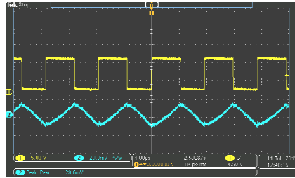
Vin=10V Vout=5V Iout=1A
