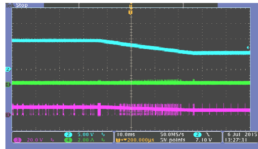
Vin=12V,Iout=0A,Vout 9V→5V
