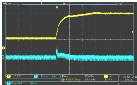
Vin=12V-40V
