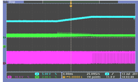
Vin=12V,Iout=2.4A,Vout 9V→5V
