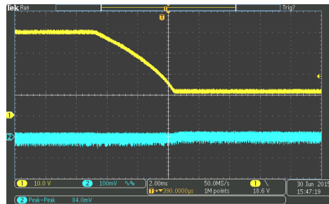
Vin=40V-12V
