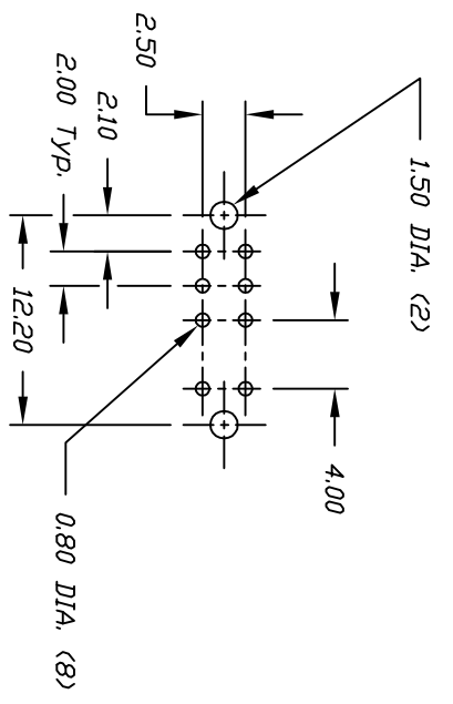
RECOMMEND P.C.B. LAYOUT
