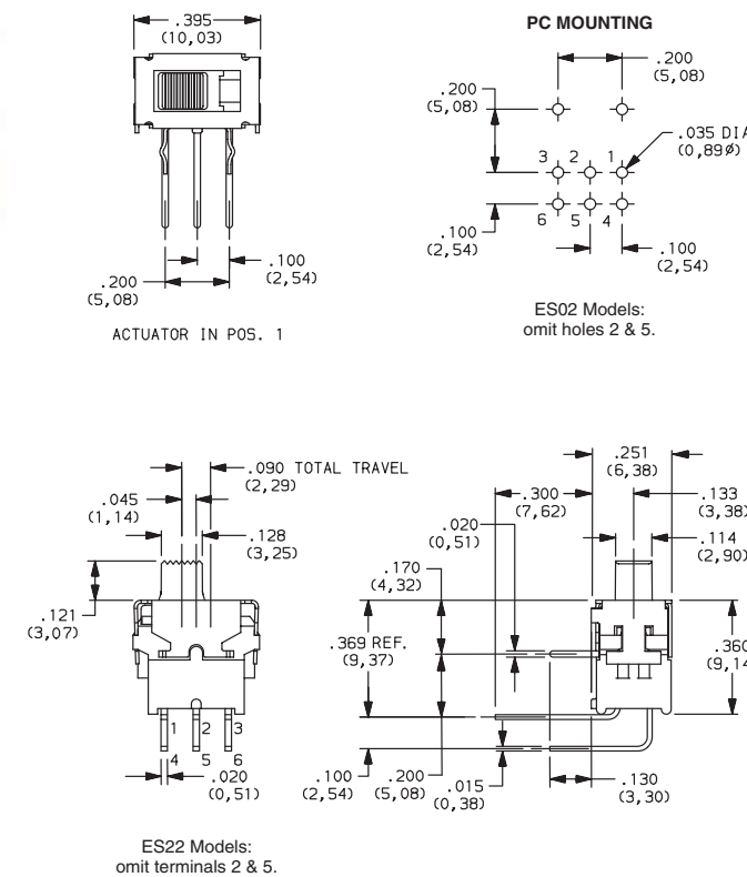
ES21MABE DPDT
