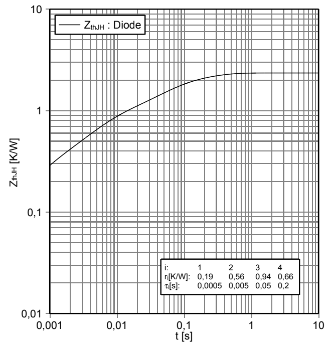
Transienter Wärmewiderstand Diode, Hochsetzsteller transient thermal impedance Diode, Boost Z_{thJH} = f(t)
