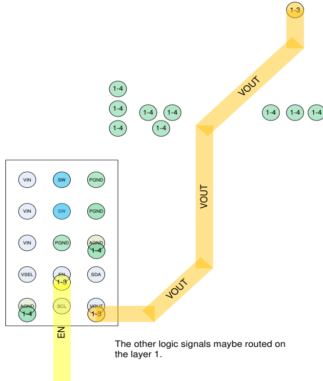
Figure 26. Layer 3
