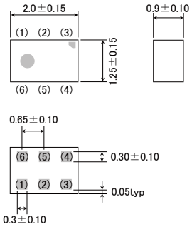
FI 212P***G* type Unit : mm
