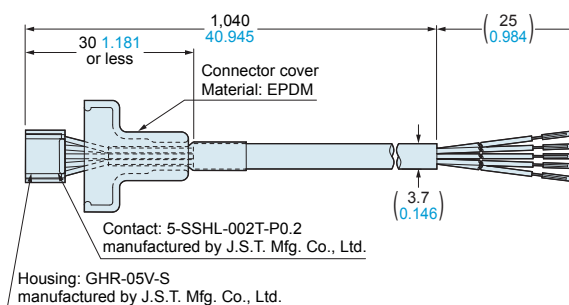
CN-F15-C1
