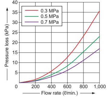
FM-216-A□2(-P)
