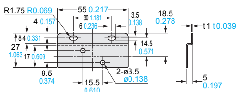
MS-FM2-1
