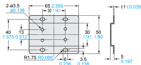
MS-FM2-2
