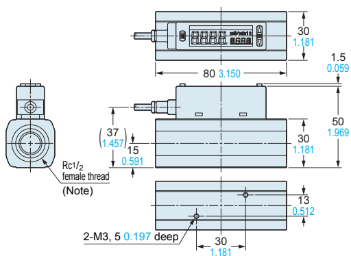
FM-2□-A□(-P)
