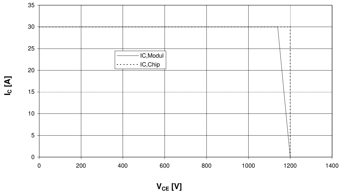
Sicherer Arbeitsbereich Wechselr. (RBSOA)
