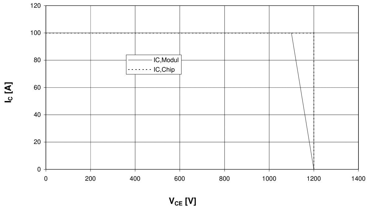
Sicherer Arbeitsbereich Wechslr. (RBSOA)
