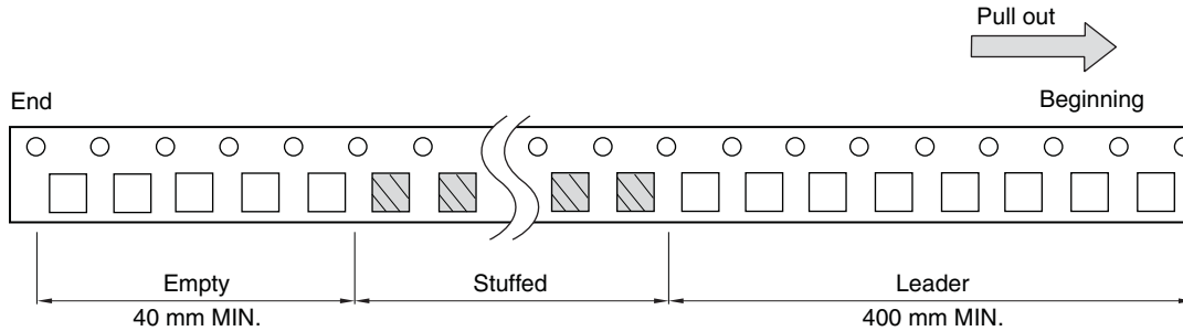
Fig. 13 Leader Tape
