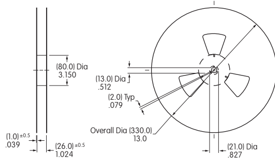
Reel Dimensions
