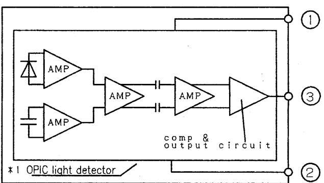
内部等価回路 Internal equivalent circuit
