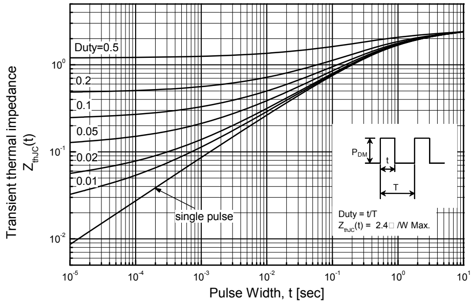
GP2M010A065F
