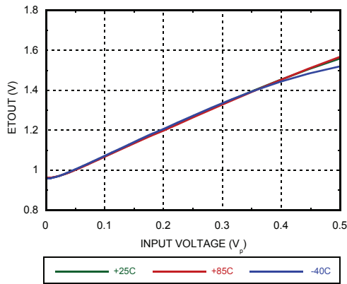
ETOUT vs. Vin with CW @ 900 MHz
