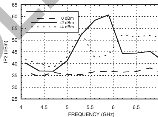
Input IP2 vs. LO Drive
