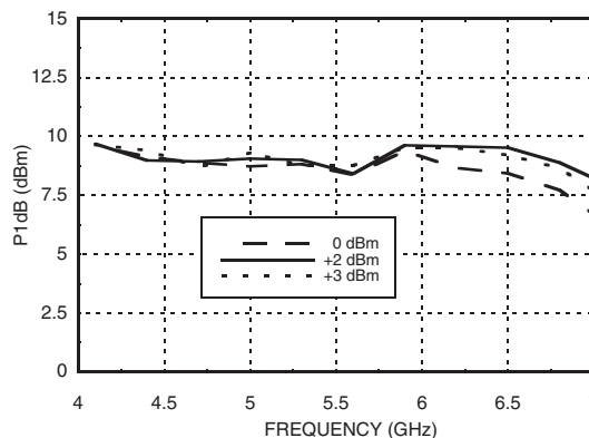
Input P1dB vs. LO Drive
