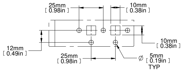
DETAIL A 10:1
